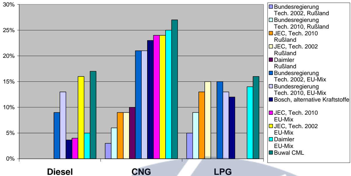
Abbildung 1, WTW-Daten zur CO 2 -Einsparung aus Literaturstellen
