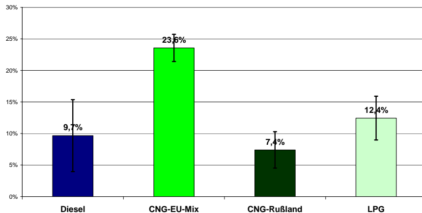
Abbildung 2, gemittelte WTW-Daten zur CO 2 -Einsparung aus Literaturstellen
