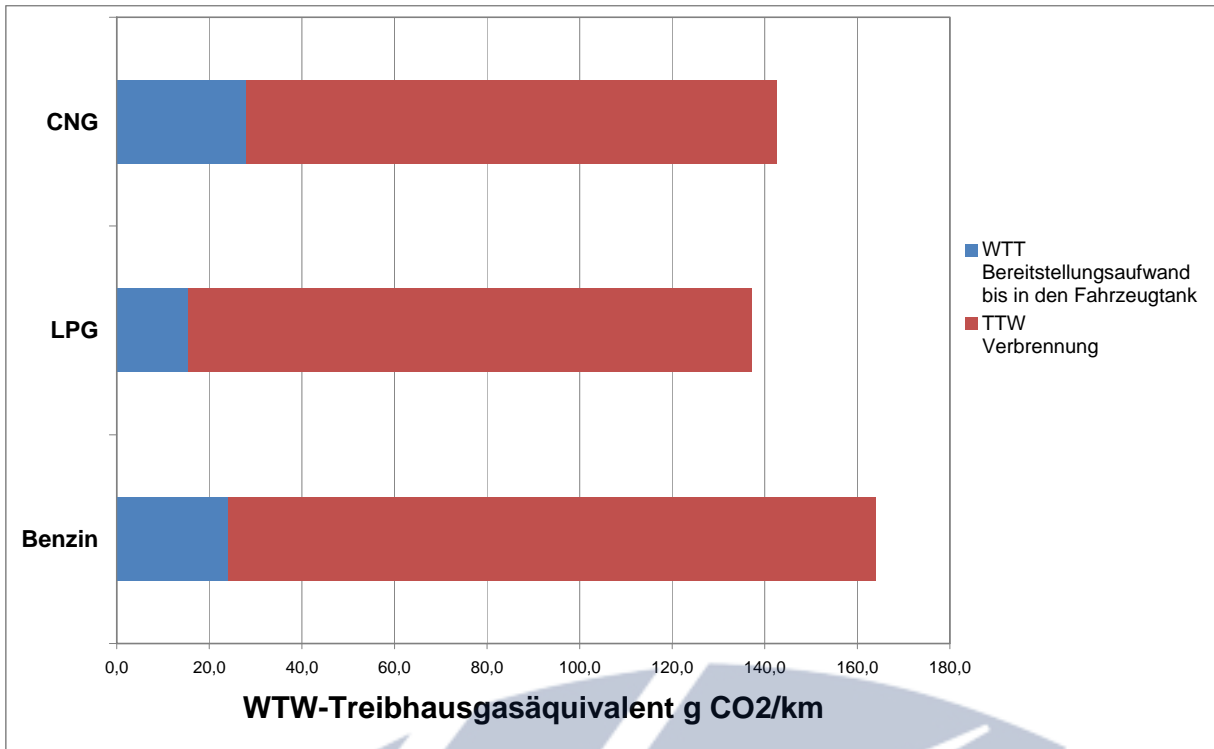
Abbildung 3, Fahrstrecken bezogenes Treibhausgasäquivalent in g CO 2 /km unter Berücksichtigung von gemittelten Fahrzeug-Typprüfwerten
