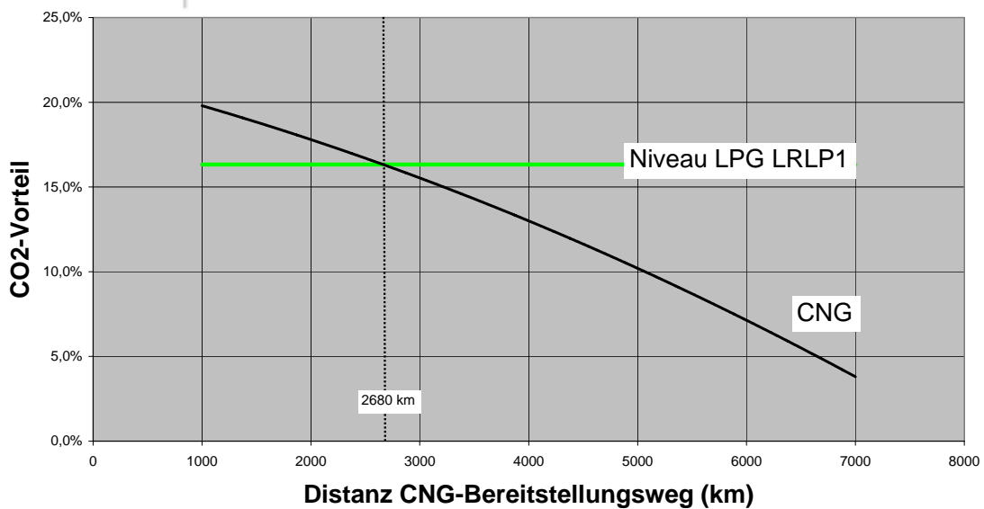
Abbildung 4, WTW- CO 2 -Vorteil bei CNG-Betrieb in Abhängigkeit vom Bereitstellungsweg
